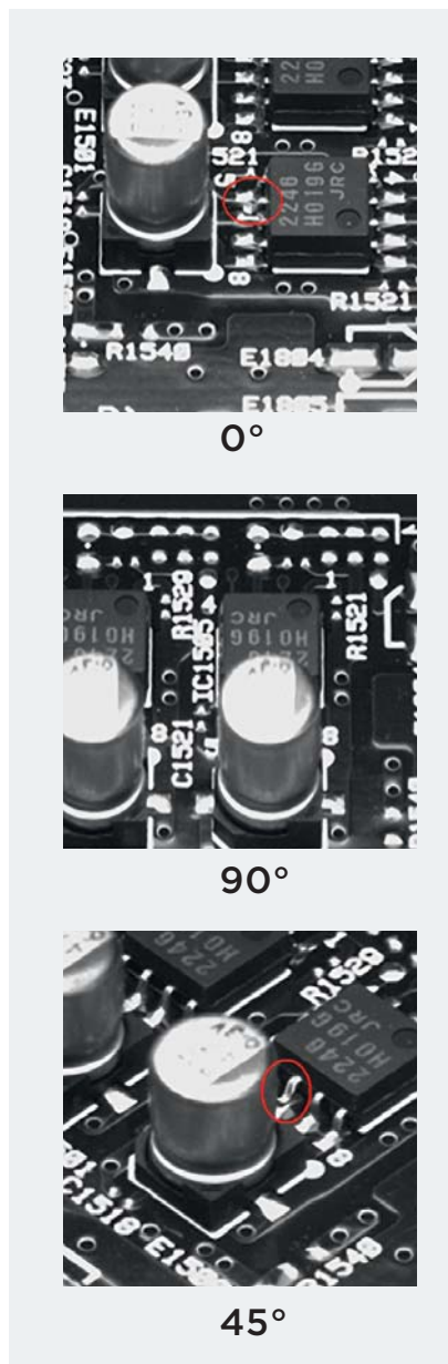
5 Дефект: отсутствие пайки вывода у компонента SO-8 под различными углами обзора
