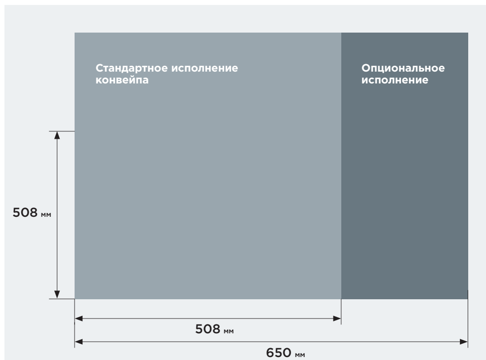
12 Стандартное и увеличенное поле S3088-flex
