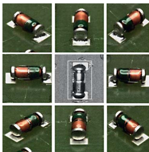
11 Компонент MELF под разными углами обзора
